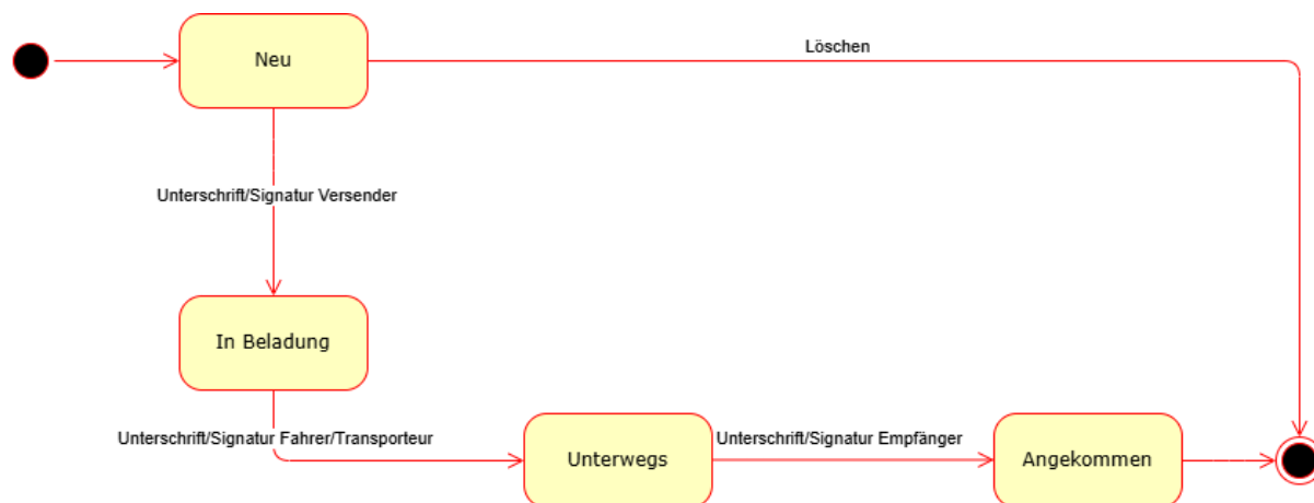
Abbildung 5: Statusmodell eCMR
